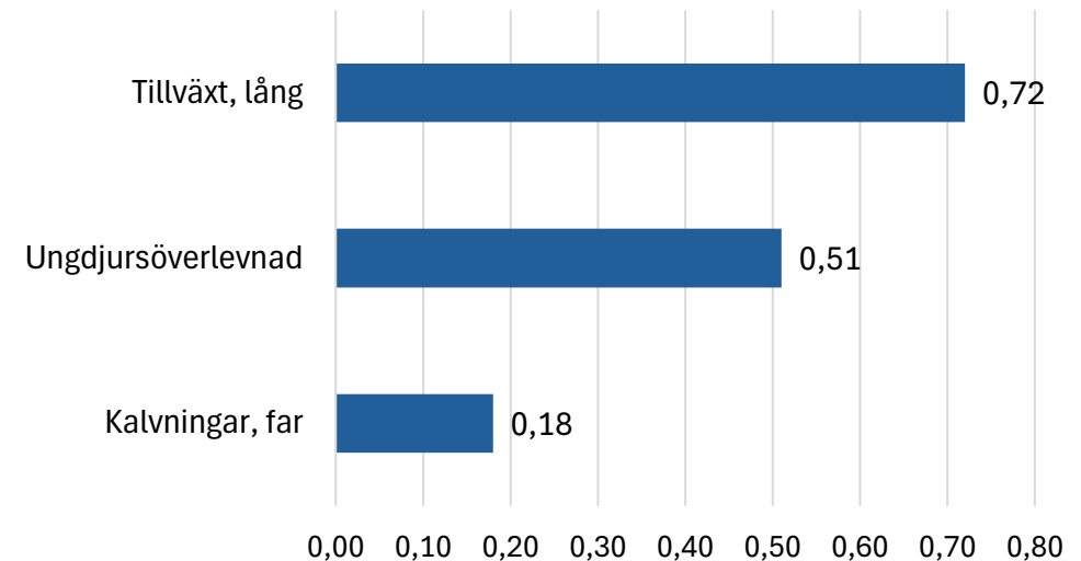
Korrelationer mellan NBDI, lång och delindex
