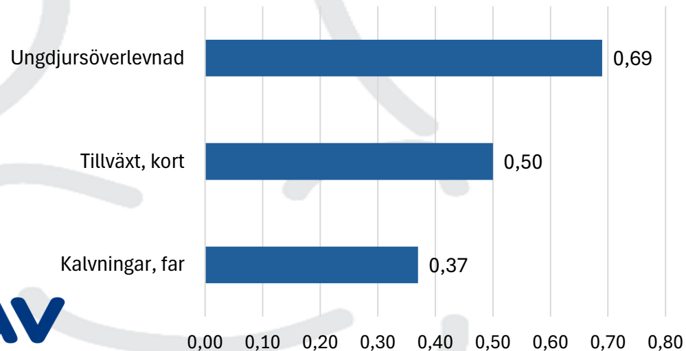
Korrelationer mellan NBDI, kort och delindex
